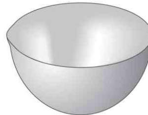
BD-2481 Ø 40 mm 15 cc Ø 60 mm 75 cc Ø 80 mm 225 cc Ø 100 mm 325 cc Ø 120 mm 500 cc
